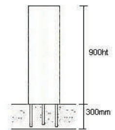
219dia S/S bollard - Inground Mnt
